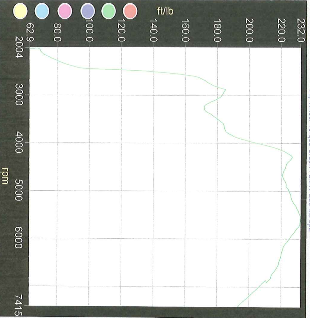
Fly Wheel Torque Graph : BMW E36 M3 3p2
