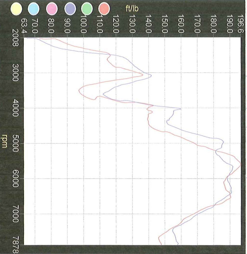
Fly Wheel Torque Graph : BMW E30 M3 2pt5
